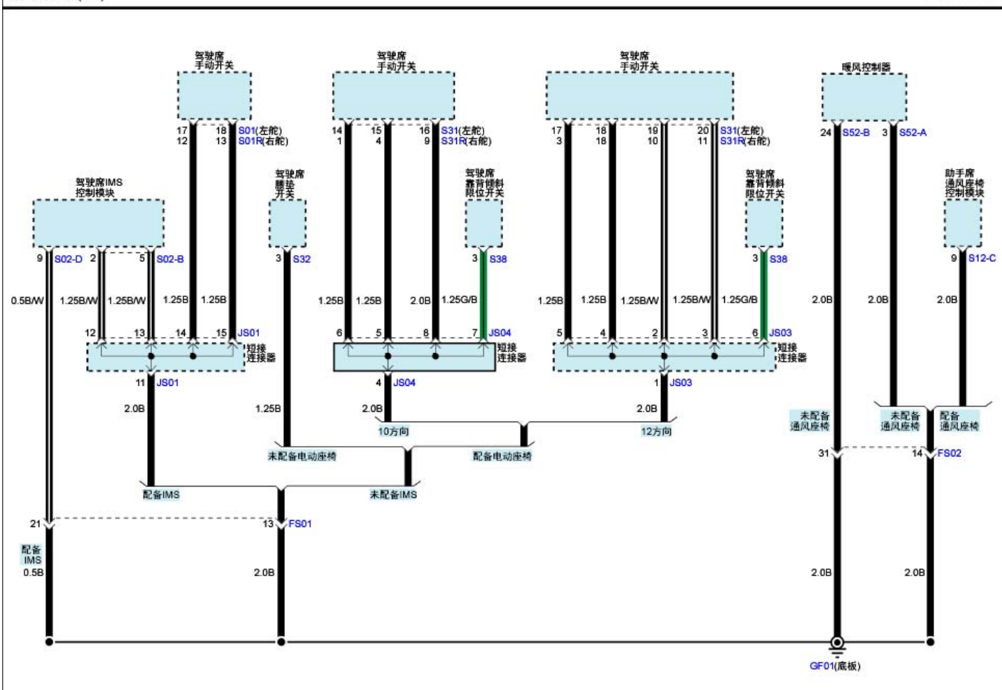
搭铁分布(10)
